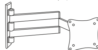
Šrouby čtyř otočných bodů s vnitřními klíčovými otvory je nutné pevně utáhnout přiloženými šestistrannými klíči.
