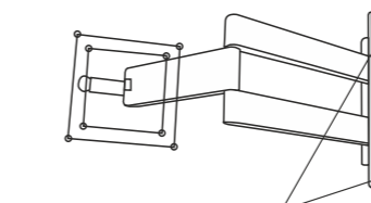
Dva otvory, určené pre pripevnenie konzoly na stenu
