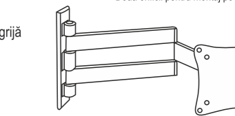
Șuruburile celor patru puncte pivotante se vor strânge strâns cu cheile hexagonale cu locaș interior anexate.
