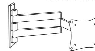
A négy forgáspont belső kulcsnyílású csavarjai a mellékelt hatlapú kulcsokkal szorossra húzandók.
